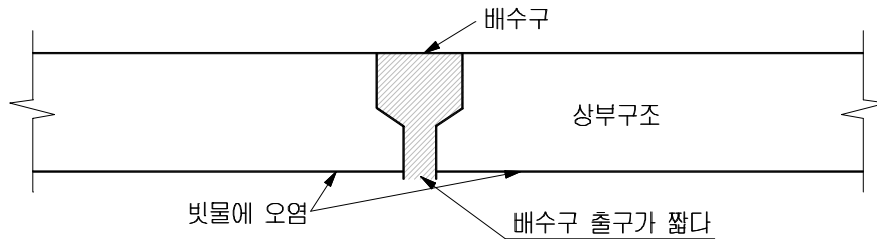
【그림 3.2.22】 배수구 길이 부족
